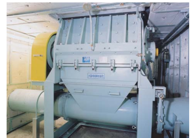
2次破砕機 乾燥機のごみをさらに細かくします。
